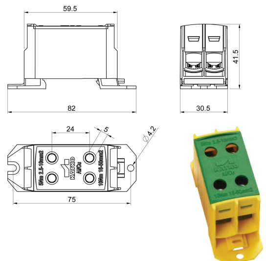
KL 2x50
