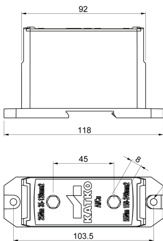
KL 1x240
