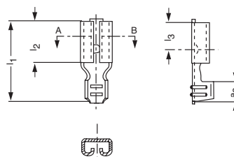
Schnitt A-B
