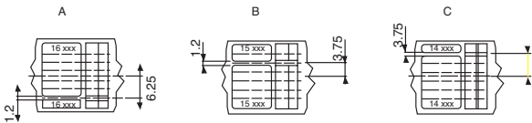
Flachsteckerwanne 2,8 x 0,8 mm
