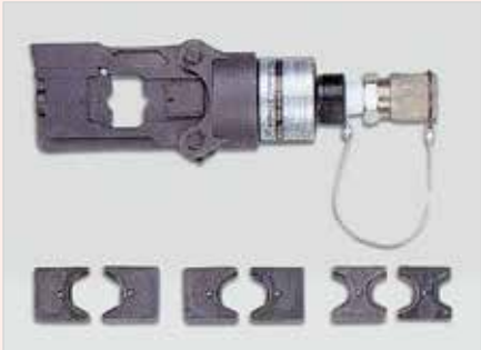
THX-185-H 1 Cabezal con matrices. Ver cuadro
