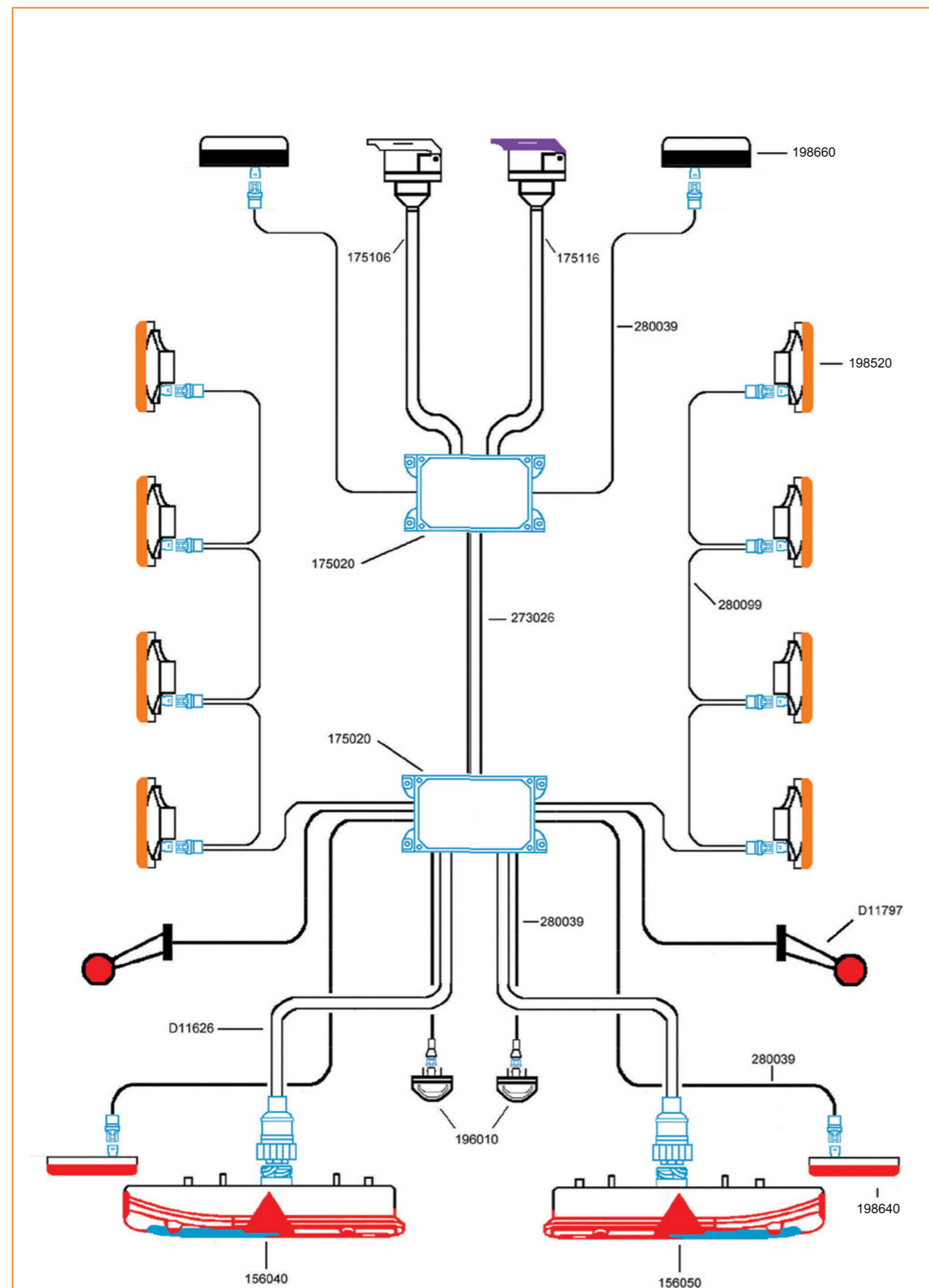
Exemple de montage - Assembly suggestion - Montagebeispiel
